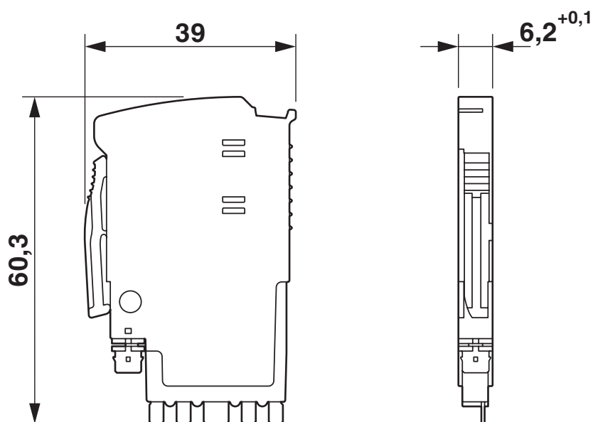
Dessin coté
