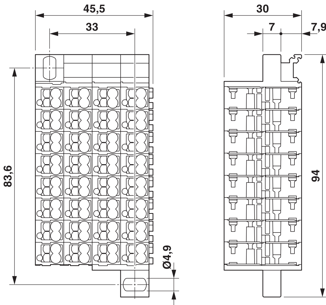
Dessin coté
