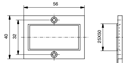
Adaptateur pour découpe: 26546843
