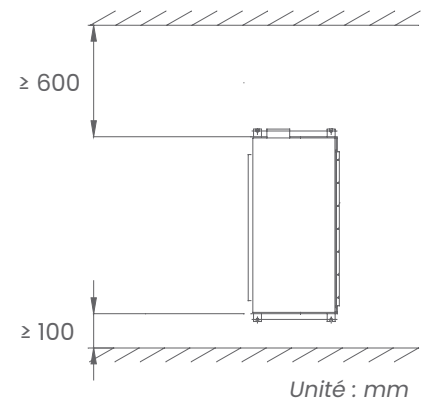
Exemple d'emplacement d'installation d'un gainable
