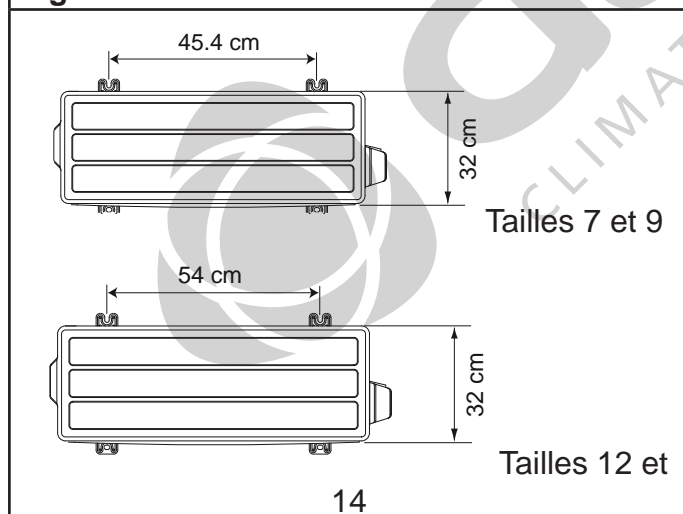
Fig. 3 - Cotes des unités extérieures
