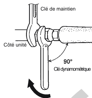
Fig. 11 - Serrage
