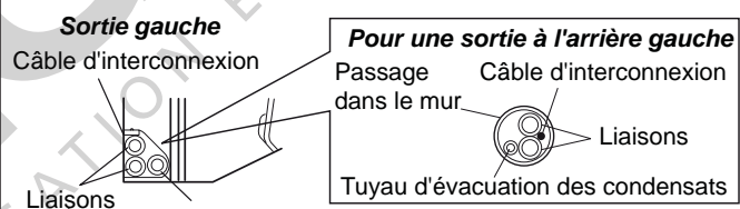
Fig. 42 - Sortie gauche ⑤ et arrière gauche ④
