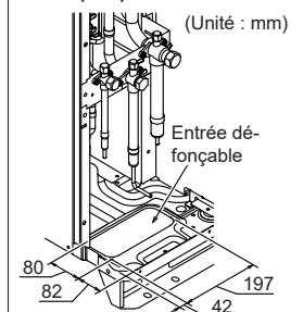
Fig. B Détail de la position de l'entrée défonçable (bas)
