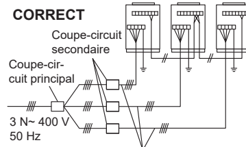
Câble d'alimentation de l'unité extérieure
