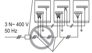
Câble d'alimentation de l'unité extérieure
