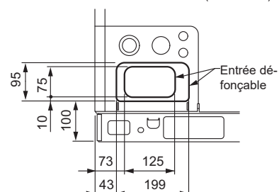
Fig. C Détail de la position de l'entrée défonçable (avant)
