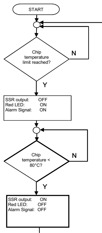
Signalisation ALARME
