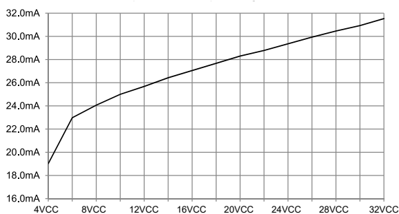
Courant d'entrée par rapport à la tension d'entrée
