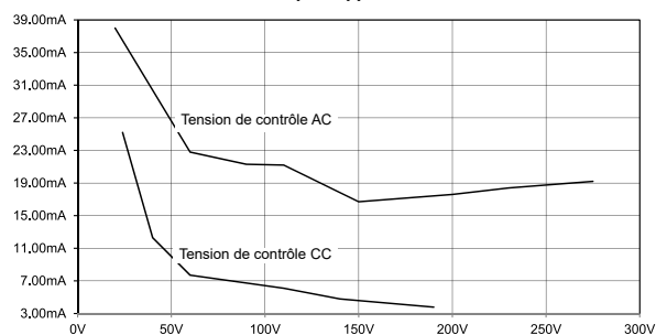
Courant d'entrée par rapport à la tension d'entrée
