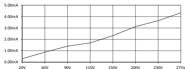
Courant d'entrée par rapport à la tension d'entrée
