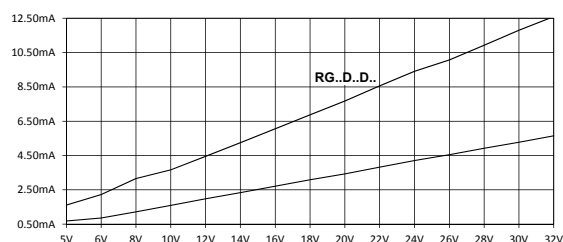
Courant d'entrée par rapport à la tension d'entrée
