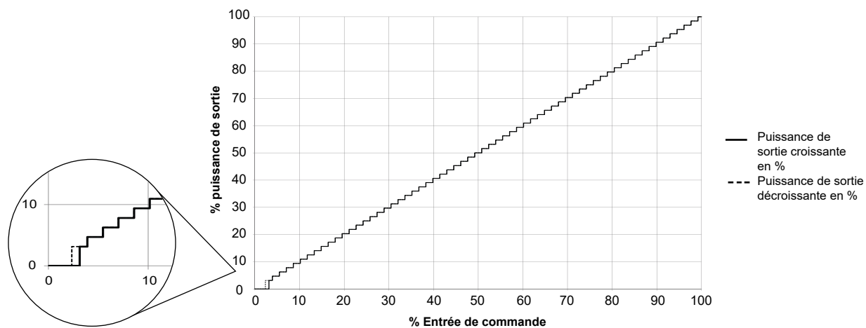
Mode de commutation complet à 4 cycles: RGC...C4
