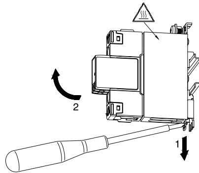
Dépose d'un relais monté sur rail DIN
