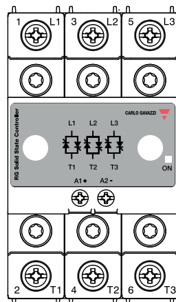
RGC2P..AA25, RGC2P..AA40 RGC3P..AA20, RGC3P..AA30
