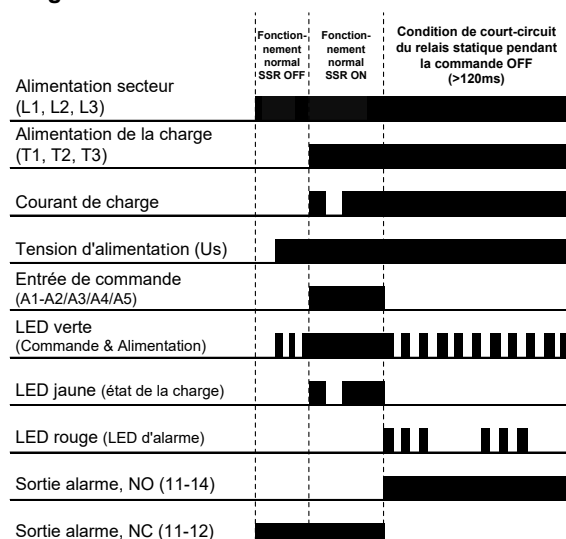
Diagramme de fonctionnement 5:
