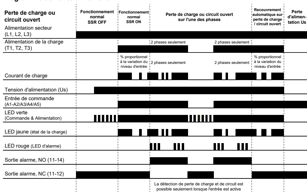
Diagramme de fonctionnement 5:
