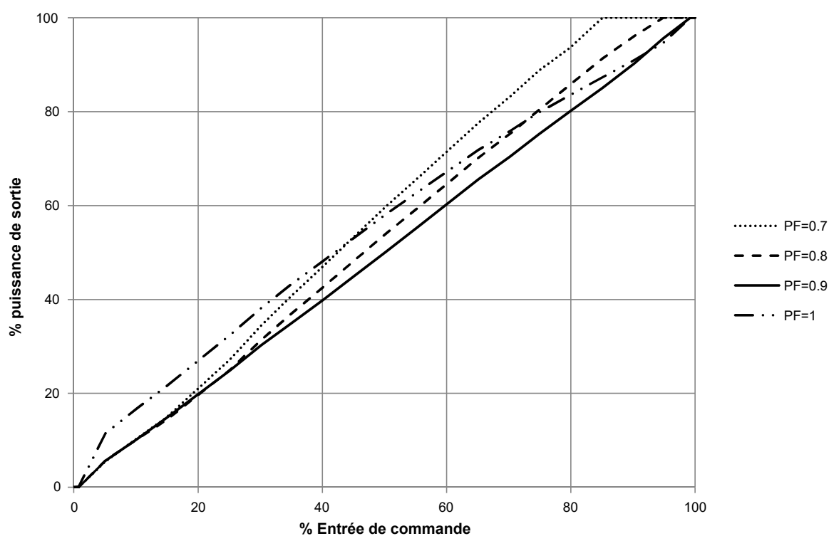
Systèmes triphasés, 4 fils
