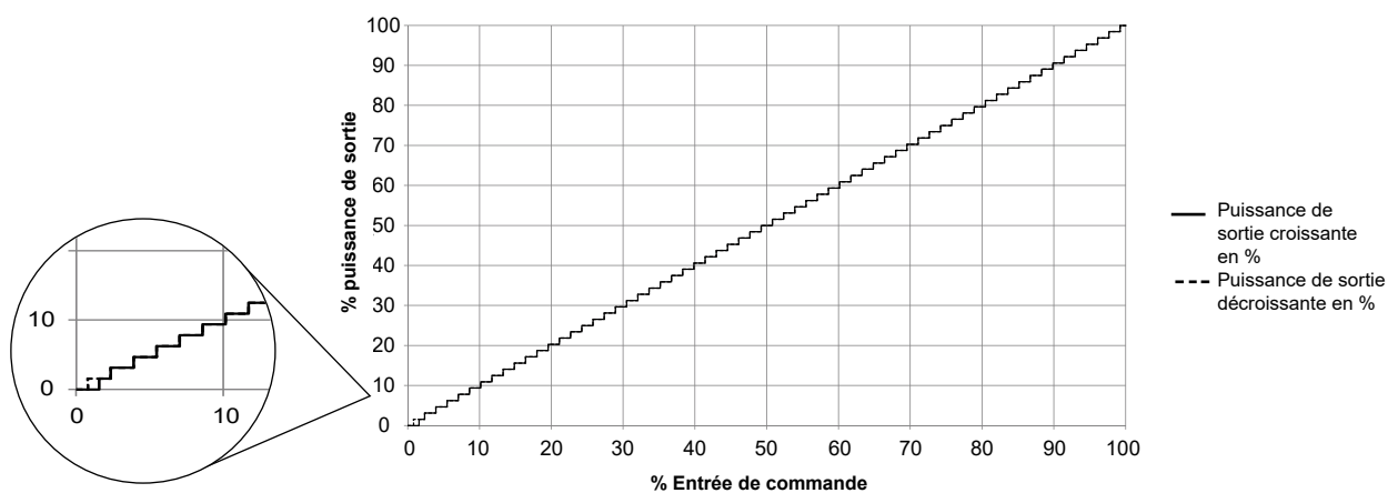
Mode de commutation complet à 1 cycle: RGC...C1
