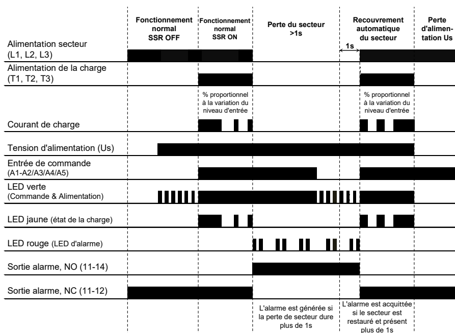
Diagramme de fonctionnement 3:
