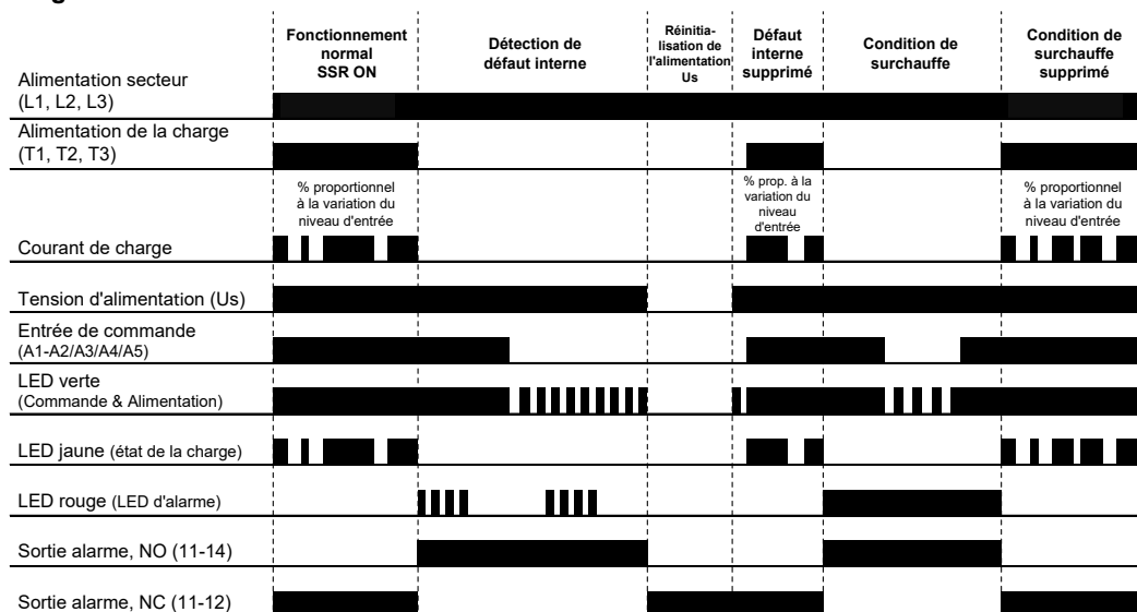
Diagramme de fonctionnement 3:
