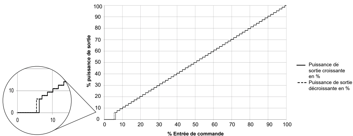
Mode de commutation complet à 16 cycles: RGC...C16
