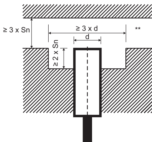
Fig. 16 Détecteur en montage non-noyable, les distances mini de montage doivent être respectées
