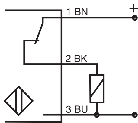
Fig. 5 PNP - NF
