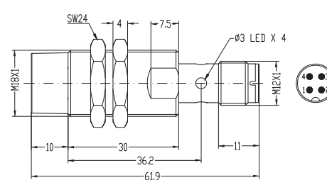
Fig. 9 Boîtier court, non noyable, connecteur
