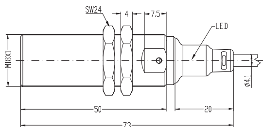
Fig. 10 Boîtier long, noyable, câble
