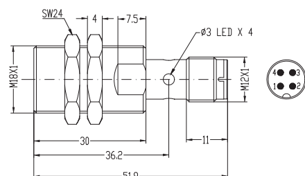
Fig. 8 Boîtier court, noyable, connecteur
