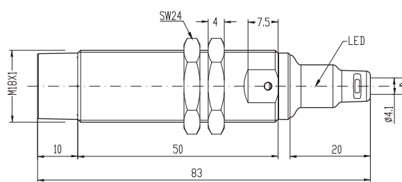
Fig. 11 Boîtier long, non noyable, câble
