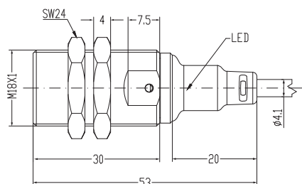
Fig. 6 Boîtier court, noyable, câble
