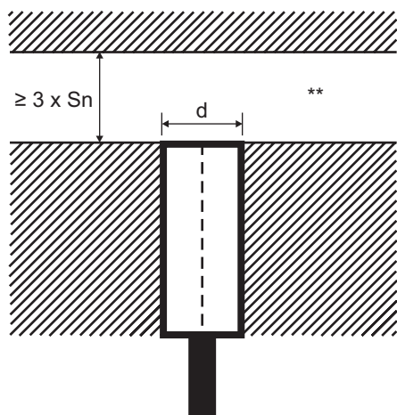
Fig. 14 Détecteur affleurant en montage noyable, les distances mini de montage doivent être respectées
