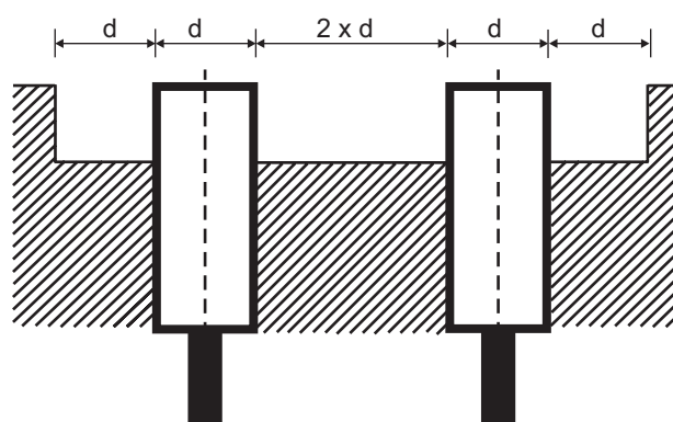
Fig. 17 Détecteurs en montage non-noyable, les distances mini de montage doivent être respectées
