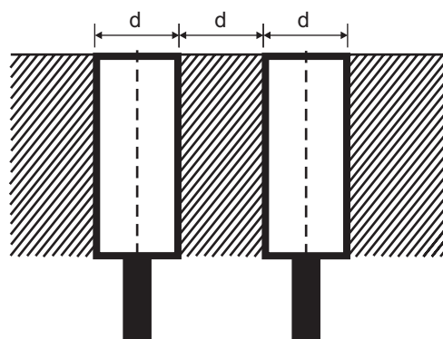
Fig. 15 Détecteur affleurant en montage noyable, les distances mini de montage doivent être respectées
