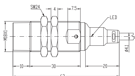
Fig. 7 Boîtier court, non noyable, câble
