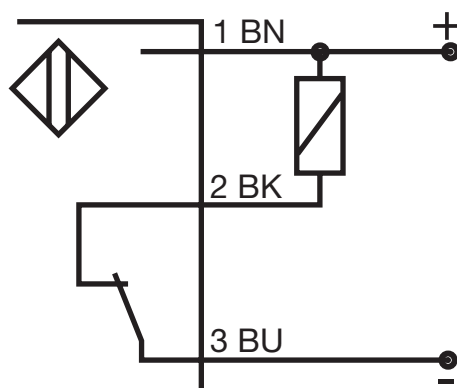
Fig. 3 NPN - NF
