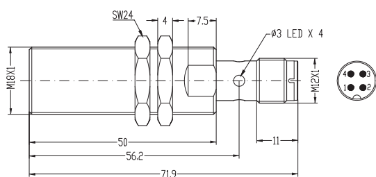
Fig. 12 Boîtier long, noyable, connecteur
