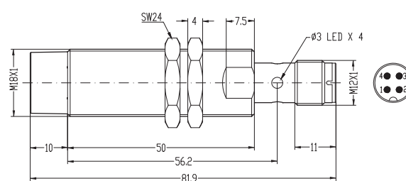
Fig. 13 Boîtier long, non noyable, connecteur
