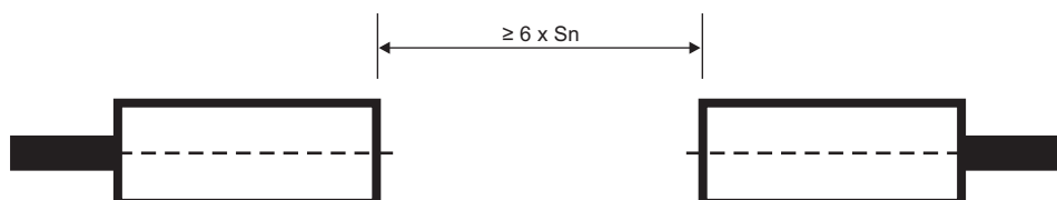
Fig. 18 Pour deux détecteurs montés en opposition, une distance mini de 6 \times S_n (distance de détection nominale) doit être respectée
