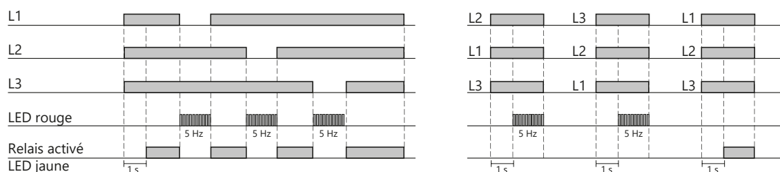
Fig. 1 Perte totale de phase, séquence de phase
