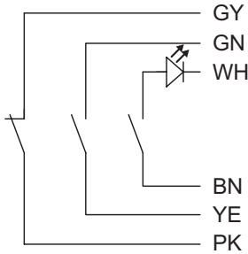
1NF + 2NO, câble avec LED
