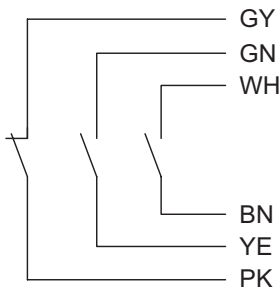
1NF + 2NO, câble
