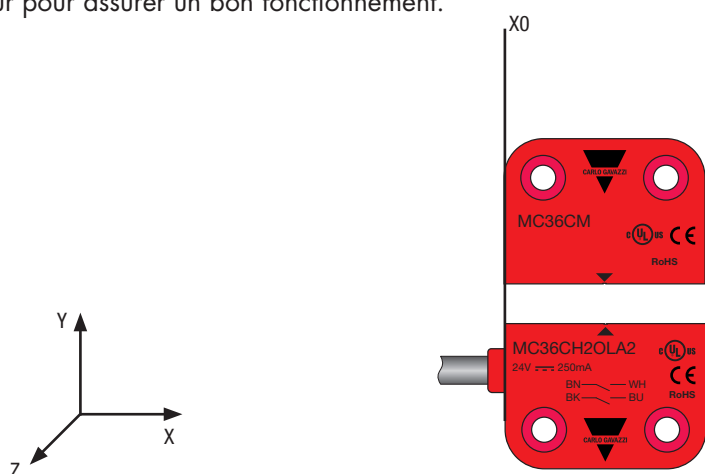
Fig. 2 - Utilisation et sens d'alignement du couple détecteur - actionneur
