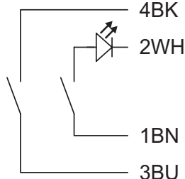
2NO, câble avec LED
