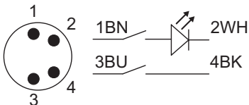
2NO, Connecteur embrochable avec LED
