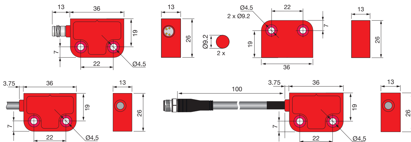
Fig. 1 - Dimensions
