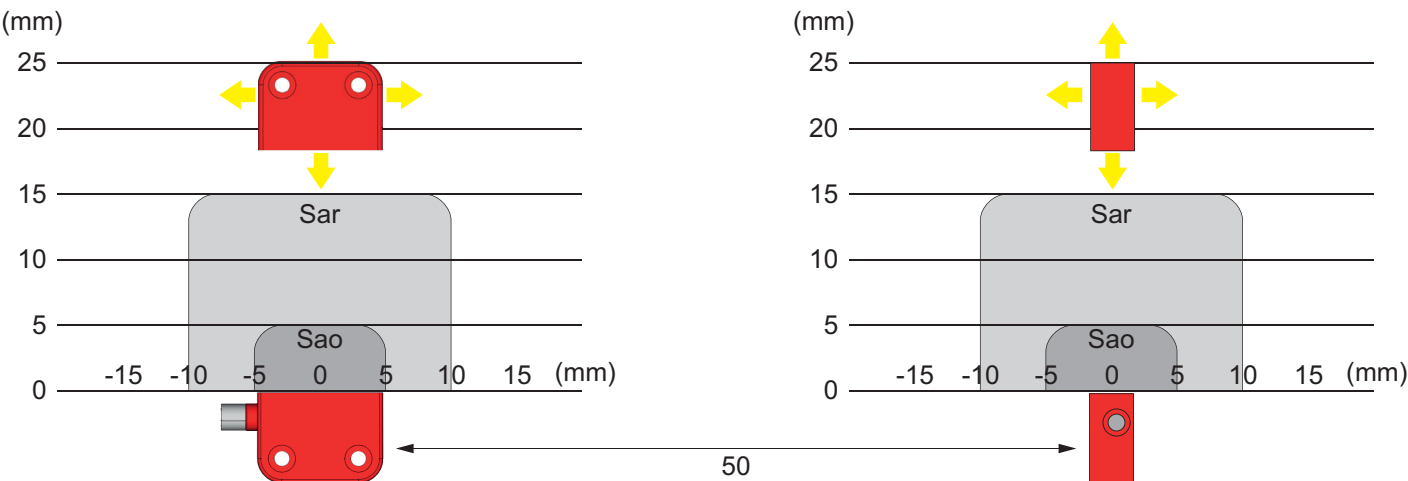
Fig. 3 - Distance
