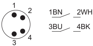
2NO, Connecteur embrochable
