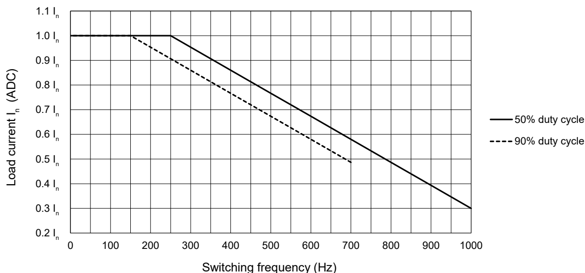
Fig. 6 Réduction de courant vs. fréquence de commutation 5
