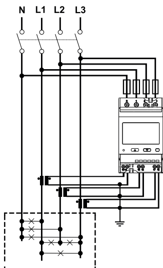
Fig. 5 Triphasé avec neutre (4 fils). MID
