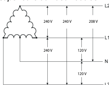
Fig. 4 Système biphasé avec neutre (3 fils)
