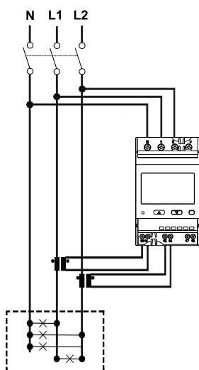
Fig. 11 Système biphasé avec neutre (3 fils)
