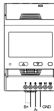
Fig. 16 Dernier appareil sur RS485
