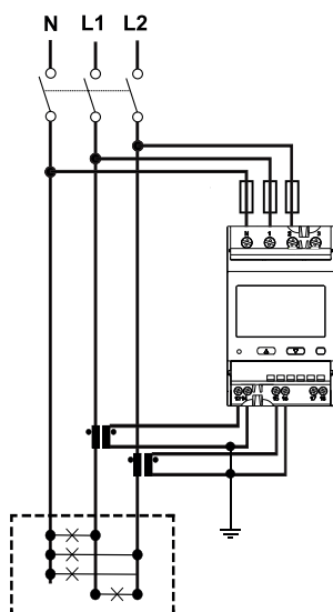
Fig. 7 Système biphasé avec neutre (3 fils)
