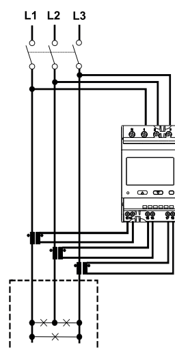
Fig. 10 Triphasé sans neutre (3 fils).
