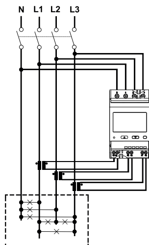
Fig. 9 Triphasé avec neutre (4 fils).
