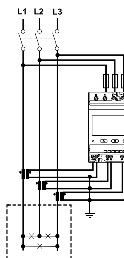
Fig. 6 Triphasé sans neutre (3 fils). MID
