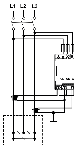
Fig. 8 Triphasé sans neutre (3 fils). MID
