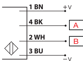
Fig. 8 NPN
