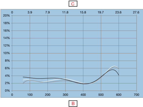
Fig. 7 Mode précision
