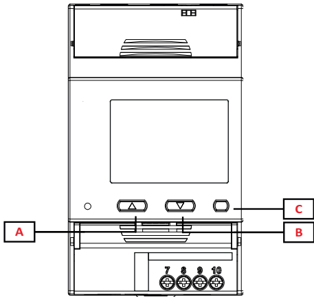
Figure 9 Façade de l'appareil
