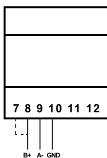
Modbus RTU: RS485 Slave (dernier appareil)
