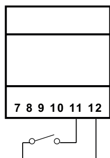
Entrée numérique
