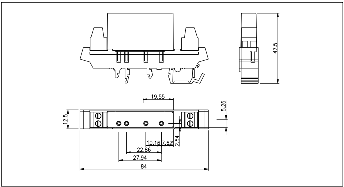
Cotes en mm, relais statique inclus
