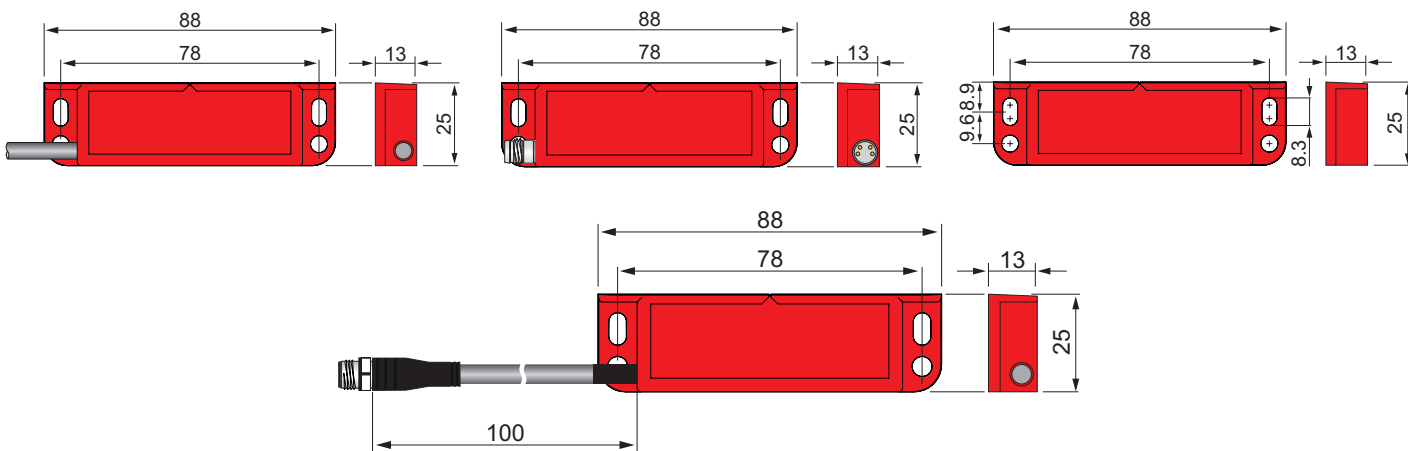
Fig. 1 - Dimensions
