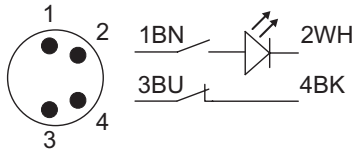
Connecteur embrochable 1NF + 1NO avec LED
