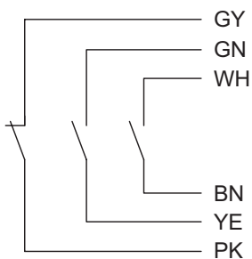
1NF + 2NO, câble
