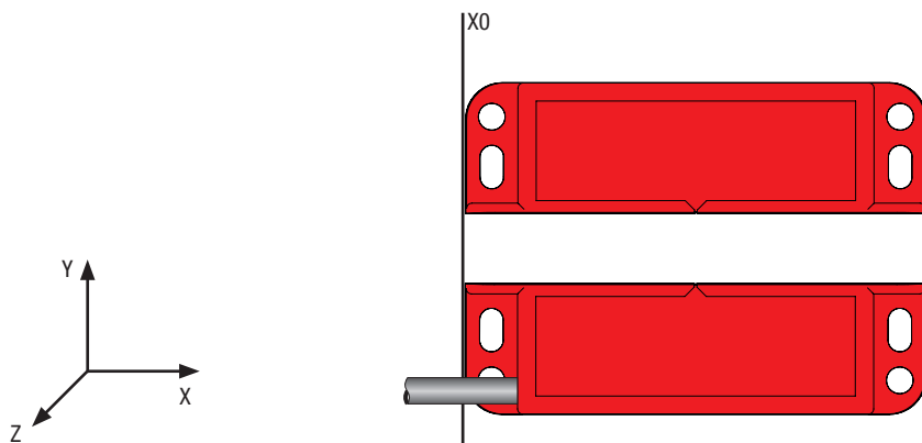
Fig. 2 - Utilisation et sens d'alignement du couple détecteur - actionneur
