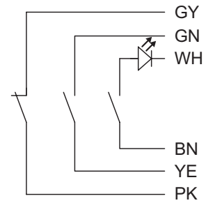
1NF + 2NO, câble avec LED
