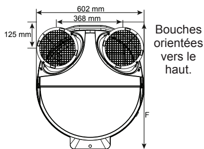
Vues de dessus
