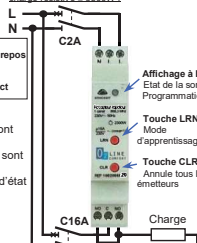
Schéma de raccordement pour charge résistive < 3500W.
