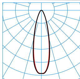
E-Line M-T LED6500-840 IP54 TX053369
