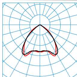
7650M-TB LED5500-840 ETDD TX040514
