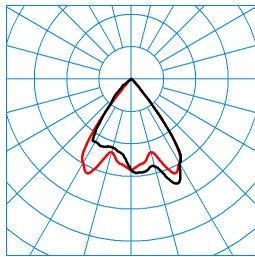
InperiaLP C05 WW-MR 1800-830 01 + DA 01 TX052067
