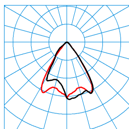
InperiaLP C05 WW-MR 1800-830 01 + RD-PC TX045526 ■ C0 - C180 ■ C90 - C270 DIN 5040: A60 UTE: 1,00 A CEN Flux Code: 86 96 99 100 100
