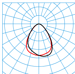
InperiaLP C05 WW-MR 1800-830 01 + DA-M 01 TX045534 ■ C0 - C180 ■ C90 - C270 DIN 5040: A50 UTE: 1,00 C CEN Flux Code: 67 91 98 100 100
