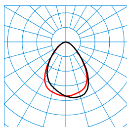
InperiaLP C05 WW-MR 1800-830 01 + DA-M 03 TX045525 ■ C0 - C180 ■ C90 - C270 DIN 5040: A50 UTE: 1,00 C CEN Flux Code: 67 91 98 100 100
