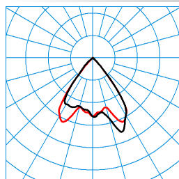
InperiaLP C05 WW-MR 1800-830 01 TX052349 ■ C0 - C180 ■ C90 - C270 DIN 5040: A60 UTE: 1,00 A CEN Flux Code: 93 100 100 100 100
