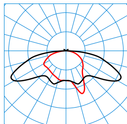
9871IA-LRA/1800-840 ET TX780517
