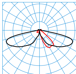
9811 AB2L/1650-740 2G1S ET TX778556
