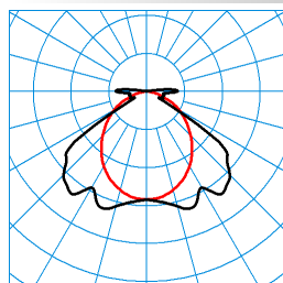
Nextrema G3 B 6000-840 +HFSB PC TX047409
