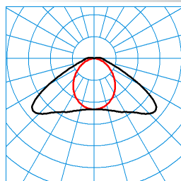
Nextrema G3 XB 6000-840 +LV TX373052
