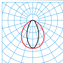
Nextrema G3 TB 6000-840 +LV PC TX371002
