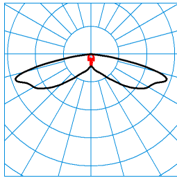
Publisca P1-SB3L/1200-740 2G1S TX047691 ■ C0 - C180 ■ C90 - C270 DIN 5040: A30 UTE: 1,00 l CEN Flux Code: 31 65 93 100 100
