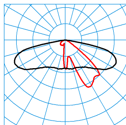
Publisca P2-AB2L-LRA/1200-730 2G1S ET (CLO initial value) TX300450
