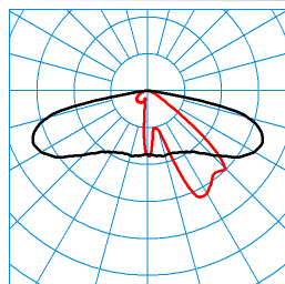
Publisca P2-AB2L-LRA/1200-730 2G1S TX047772
