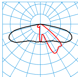
Publisca P2-AB2L-LRA/1200-730 2G1S ET (CLO end value) TX300450
