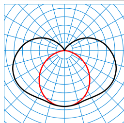
6651 S LED1100-840 ET TX773627
