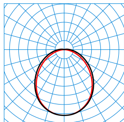
3331 G2 D3 TS LED3000-830 ETDD 03 TX771374
