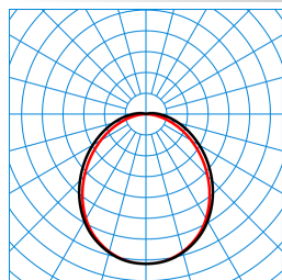
3331 G2 D3 TS LED3700-840 ET 03 TX771399
