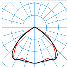
7650 LightP G2 B-B-B 8000-840 ETDD 05 TX808781
