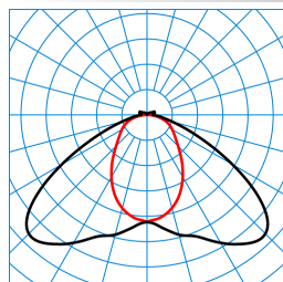
7640XB LED8000-865 ET TX808663
