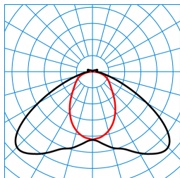
7640XB LED8000-830 ET TX829914
