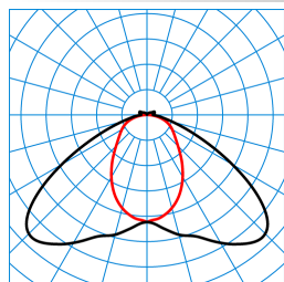
7640XB LED4000-830 ETDD 05 TX783230
