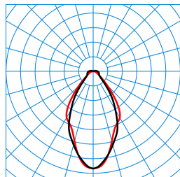
7640T LED10000-865 ET TX783437
