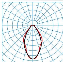
7640T LED4000-865 ET 03 TX829995
