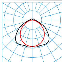
C-Line PA-TB LED4000-840 TX055360
