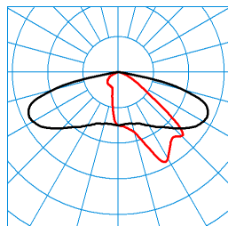
Jovie 50-AB2L-LRA/3200-730 4G1 ET (CLO initial value) TX301323 DIN 5040: A30 UTE: 1,00 G CEN Flux Code: 34 71 96 100 100 ■ C0 - C180 ■ C90 - C270
