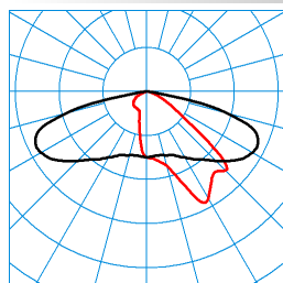
Jovie 50-AB2L-LRA/3200-730 4G1 ET TX068564 DIN 5040: A30 UTE: 1,00 G CEN Flux Code: 34 71 96 100 100 ■ C0 - C180 ■ C90 - C270
