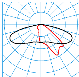
Jovie 50-AB2L-LRA/3200-730 4G1 ET (CLO end value) TX300456 DIN 5040: A30 UTE: 1,00 G CEN Flux Code: 34 71 96 100 100 ■ C0 - C180 ■ C90 - C270
