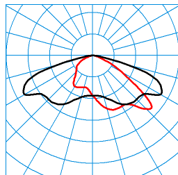
Jovie 70-AB7L-LRA/16500-730 18G1 ET (CLO end value) TX300780 ■ C0 - C180 ■ C90 - C270 DIN 5040: A30 UTE: 1,00 G CEN Flux Code: 35 72 97 100 100
