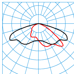
Jovie 70-AB7L-LRA/16500-730 18G1 ET (CLO initial value) TX300671 ■ C0 - C180 ■ C90 - C270 DIN 5040: A30 UTE: 1,00 G CEN Flux Code: 35 72 97 100 100
