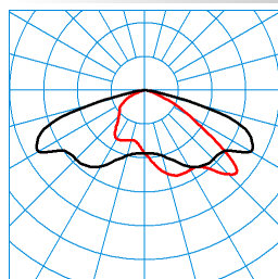
Jovie 70-AB7L-LRA/16500-730 18G1 ET TX068629 ■ C0 - C180 ■ C90 - C270 DIN 5040: A30 UTE: 1,00 G CEN Flux Code: 35 72 97 100 100
