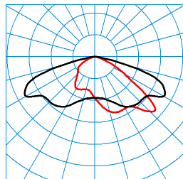
Jovie 70-AB7L-LRA/24000-730 24G1 ET (CLO end value) TX300962 ■ C0 - C180 ■ C90 - C270 DIN 5040: A30 UTE: 1,00 G CEN Flux Code: 35 73 97 100 100
