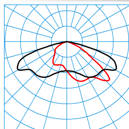
Jovie 70-AB7L-LRA/24000-730 24G1 ET TX068638 ■ C0 - C180 ■ C90 - C270 DIN 5040: A30 UTE: 1,00 G CEN Flux Code: 35 73 97 100 100
