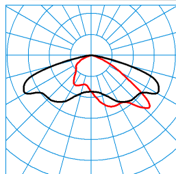
Jovie 70-AB7L-LR/10000-730 8G1 ET TX068600 DIN 5040: A30 UTE: 1,00 G CEN Flux Code: 34 71 96 100 100 ■ C0 - C180 ■ C90 - C270
