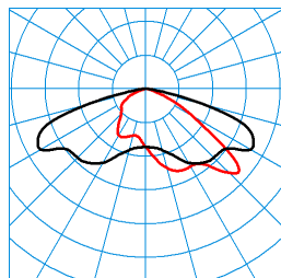
Jovie 70-AB7L-LR/10000-730 8G1 ET (CLO initial value) TX300186 DIN 5040: A30 UTE: 1,00 G CEN Flux Code: 34 71 96 100 100 ■ C0 - C180 ■ C90 - C270
