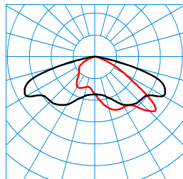
Jovie 70-AB7L-LR/10000-730 8G1 ET (CLO end value) TX300327 DIN 5040: A30 UTE: 1,00 G CEN Flux Code: 34 71 96 100 100 ■ C0 - C180 ■ C90 - C270
