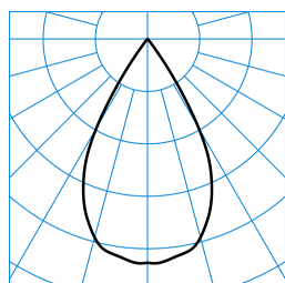
E-Line 7651 B.VEO RFS-VFL 05 30-835 J16 ET L37 01 (150) ■ C0 - C180 TX576906
