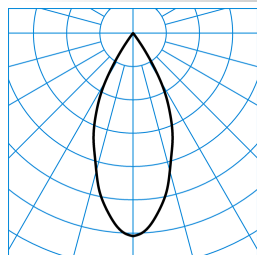
E-Line 7651 B.VEO RFS-WFL 05 30-835 J16 ET L37 01 (150) ■ C0 - C180 TX576907
