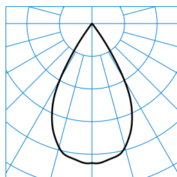
E-Line 7651 B.VEO RFS-VFL 05 30-835 J16 ET L37 01 (225) TX804985 ■ C0 - C180
