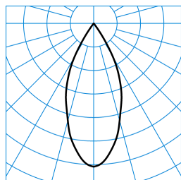
E-Line 7651 B.VEO RFS-WFL-c 05 30-835 J16 ET L37 01 (150) ■ C0 - C180 TX576911
