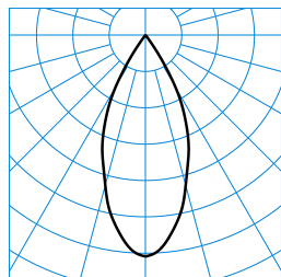
E-Line 7651 B.VEO RFS-WFL 05 30-835 J16 ET L37 01 (225) ■ C0 - C180 TX805014
