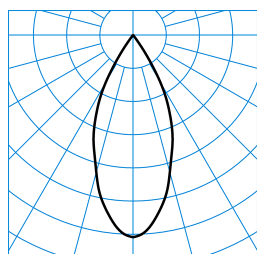
E-Line 7651 B.VEO RFS-WFL-c 05 30-835 J16 ET L37 01 (225) ■ C0 - C180 TX805029
