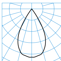
E-Line 7651 B.VEO RFS-VFL 05 40-EW J10 ET L37 05 (150) ■ C0 - C180 TX577089
