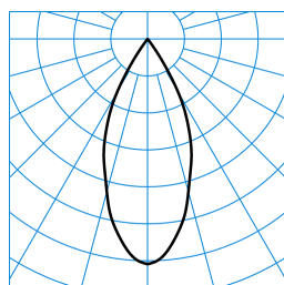
E-Line 7651 B.VEO RFS-WFL-c 05 40-EW J10 ET L37 05 (150) ■ C0 - C180 TX577094
