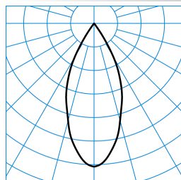
E-Line 7651 B.VEO RFS-WFL 05 40-EW J10 ET L37 05 (150) ■ C0 - C180 TX577090
