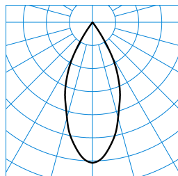
E-Line 7651 B.VEO RFS-WFL 05 40-EW J10 ET L37 05 (225) ■ C0 - C180 TX805023
