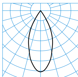
E-Line 7651 B.VEO RFS-WFL-c 05 40-EW J10 ET L37 05 (225) ■ C0 - C180 TX805037
