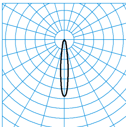
E-Line 7751 B.VEO RFS-SP 05 20-EW J10 ET L37 01 ■ C0 - C180 TX095540 DIN 5040: A80 UTE: 0,81 A CEN Flux Code: 100 100 100 100 81
