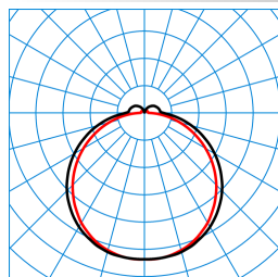
7651 LightP OTR 80-830ETDD L75 05 (150) TX557203
