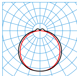
7651 LightP OTR 80-830ETDD L75 05 (225) TX557043
