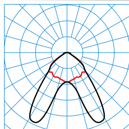
7651 LightP DA-B-DA 65-830ET L75 01 (150) TX557820
