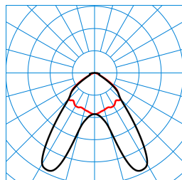
7651 LightP DA-B-DA 65-830ET L75 01 (225) TX558063
